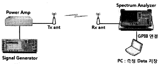
그림 2. CW 측정 시스템
