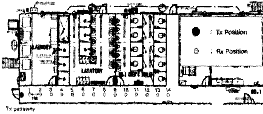
그림 4. 중앙복도에서의 측정지점
