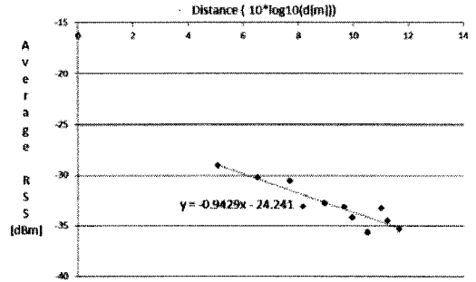
그림 9. 측정거리에 따른 수신 파워 및 결과에 따른 추세선 (체력 단련 실-가장자리)
