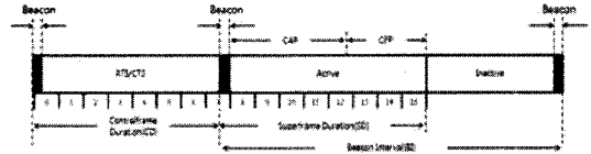
그림 4. 개선한 비콘 프레임 코디네이터 Fig. 4. Improve Beacon Frame Coordinator
