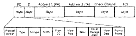
그림 6. 24비트 확장형 RTS Fig. 6. 24bit Expansion RTS
