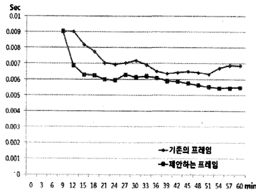
그림 12. 전체 네트워크의 평균 지연시간 (sec) Fig. 12. Average Delay of a Total Network (sec)
