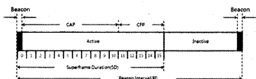
그림 1. 비콘 프레임 Fig. 1. Beacon Frame
