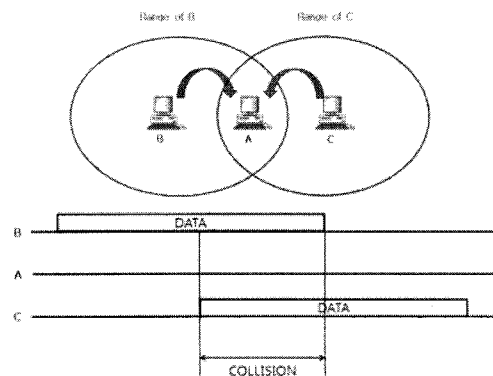
그림 2. 숨겨진 단말 문제 Fig. 2. Hidden Node Problem
