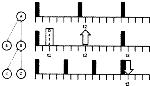
그림 3. 전송 지연 문제 Fig. 3. Transfer Delay Problem
