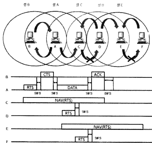
그림 5. False Node Problem Fig. 5. False Node Problem
