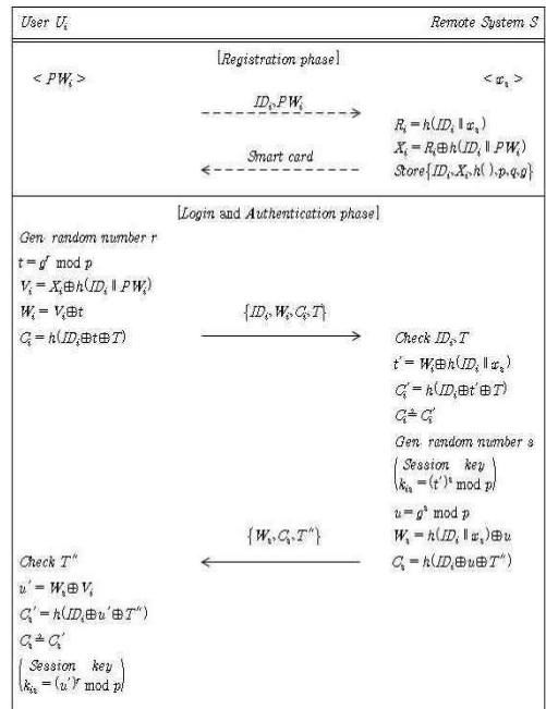
그림 1. 제안한 인증 스킴 Fig 1. The our proposed scheme
