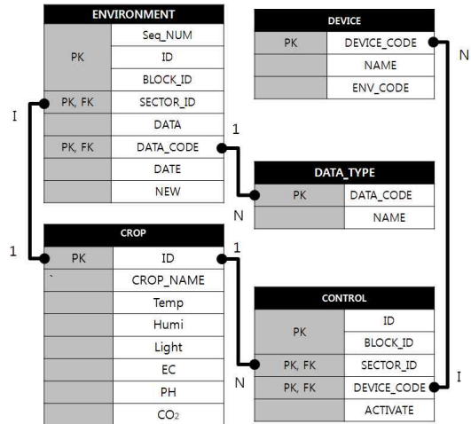
그림 8. 데이터베이스 스키마 Fig. 8. DataBase Schema
