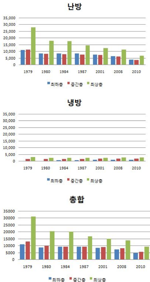
그림 4. 냉·난방 부하 변화추이
