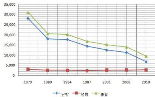
그림 3. 층에 따른 연도별 에너지 요구량 변화
