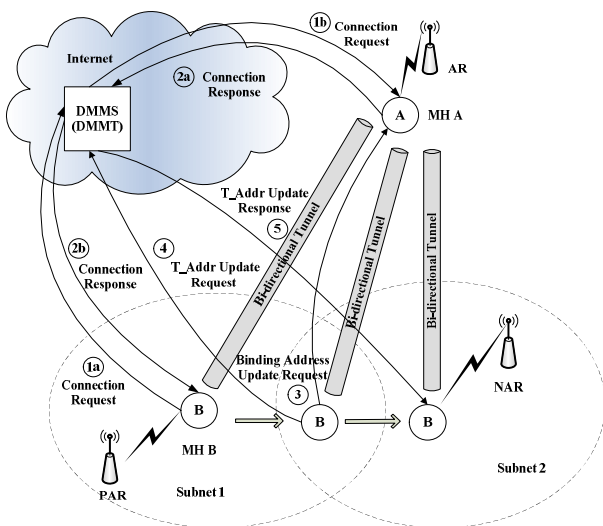
그림 2. SMMP 이동성 관리의 핸드오버 동작 Fig. 2. Handover operations of mobility management of SMMP.
