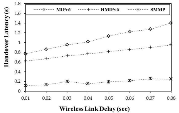
그림 5. 무선 링크 지연에 따른 핸드오버 지연시간의 영향 Fig. 5. Impact of wireless link delay on handover latency.
