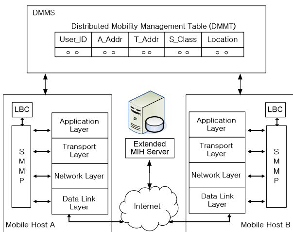
그림 1. SMMP 구조 Fig. 1. SMMP architecture.
