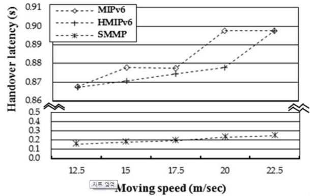
그림 6. 이동 호스트의 속도변화에 따른 핸드오버 지연시간의 변화 Fig. 6. Changes of handover latency due to change of moving speed of mobile host.
