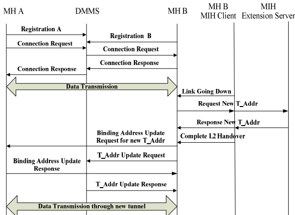
그림 3. SMMP의 시그널링 흐름 다이어그램 Fig. 3. Signaling Flow Diagram of SMMP.
