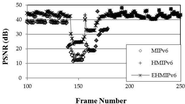
그림 8. 핸드오버하는 동안의 PSNR의 변화 Fig. 8. PSNR changes during handover.
