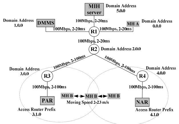
그림 4. 시뮬레이션 토폴로지 및 파라미터 Fig. 4. Simulation topology and parameters.
