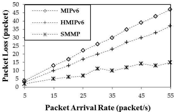
그림 7. 패킷 도착율의 변화에 대한 패킷 손실 Fig. 7. Packet loss due to changes of packet arrival rate.
