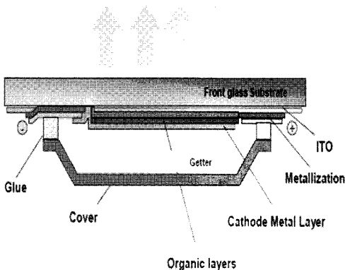
그림 1. OLED의 구조 및 OLED 패널 개념도
