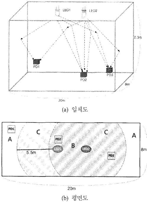
그림 1. 실내 VLC 송수신 환경의 예
