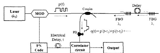
그림 1. 코드분할 다중방식 센서 네트워크 구성도
