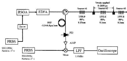
그림 4. 실험 구성도
