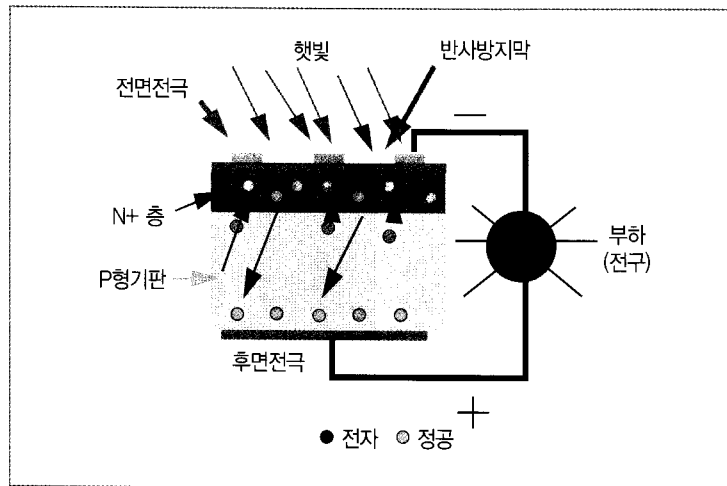
[그림 1] 태양광발전의 발전원리
