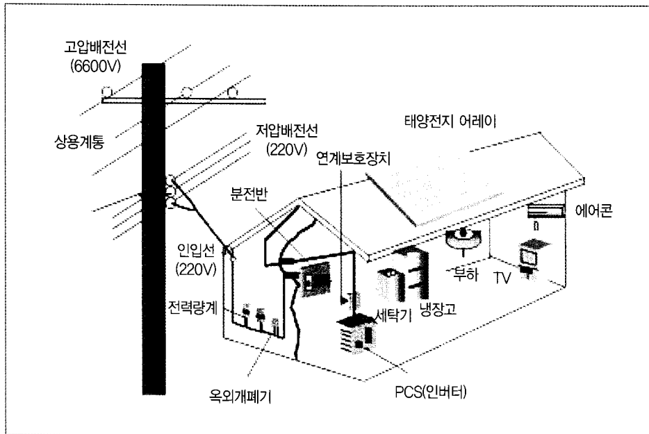
[그림 3] 태양광발전시스템의 구성도
