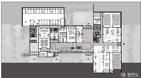
1층 평면도
