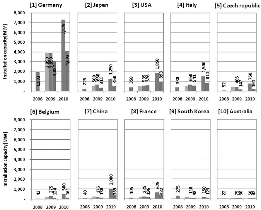
[그림 6] TOP10 국가별 2008/2009/2010(예측) PV 수요량
