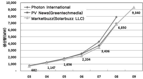
[그림 1] 태양전지 생산량 추이
