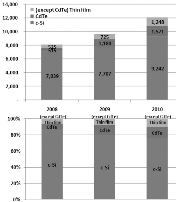
[그림 2] 태양전지 기술별 생산량 & 점유율 추이
