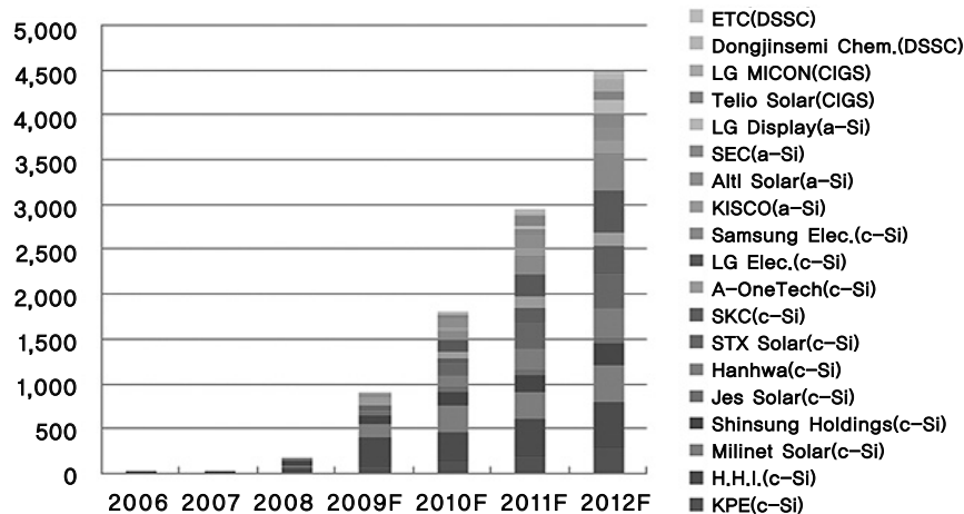
[그림 9] 국내 태양전지 생산시설용량 추이
