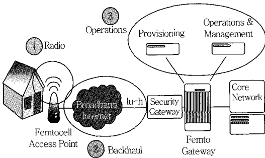
(그림 2) 펜토셀 기본 시스템 구성
