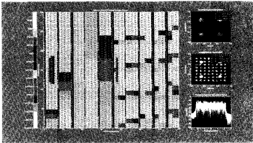
(그림 10) 4명 사용자의 LTE DL Tx RB Allocation
