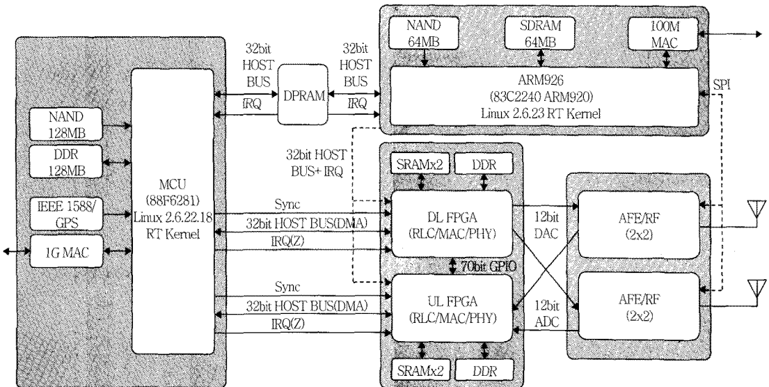
(그림 6) LTE 펌토셀 플랫폼
