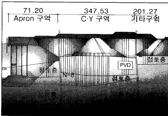
연약지반개량
