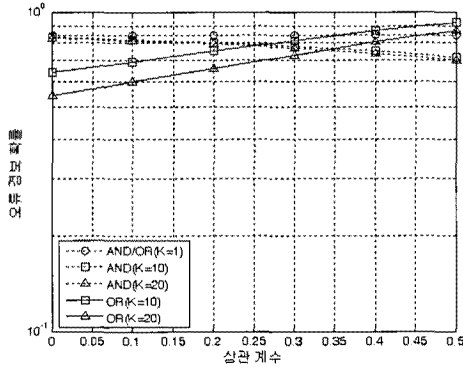
그림 2. 상관 계수에 따른 오류 정보 확률
