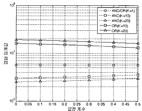
그림 1. 상관 계수에 따른 검파 임계값
