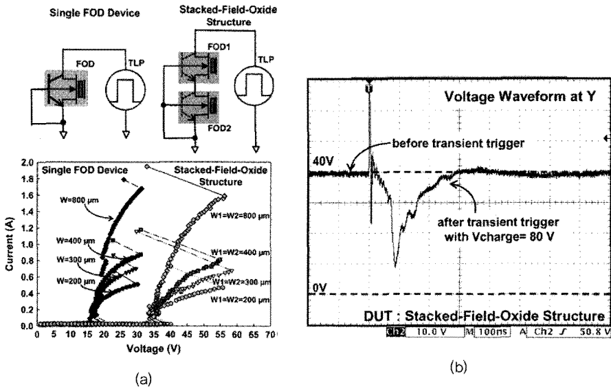
<그림 12> FOD Stack의 (a)TLP-IV 특성, (b)TLU 특성
