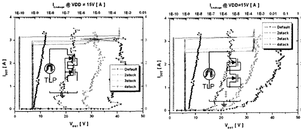
<그림 11> GGNMOS Stack의 TLP-IV 특성
