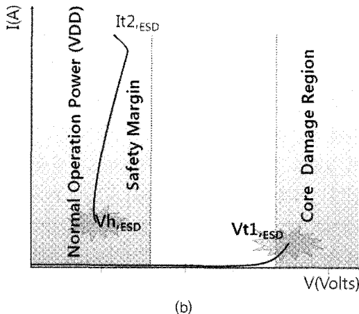
〈그림 3〉 (a) GGNMOSFET의 불균일한 트리거 효과에 따른 ESD 감내특성 감소 특성, (b)SCR의 높은 트리거 전압과 낮은 홀딩 전압 특성
