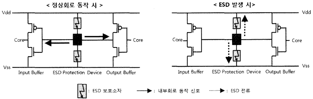
<그림 1> ESD 보호 회로의 개념
