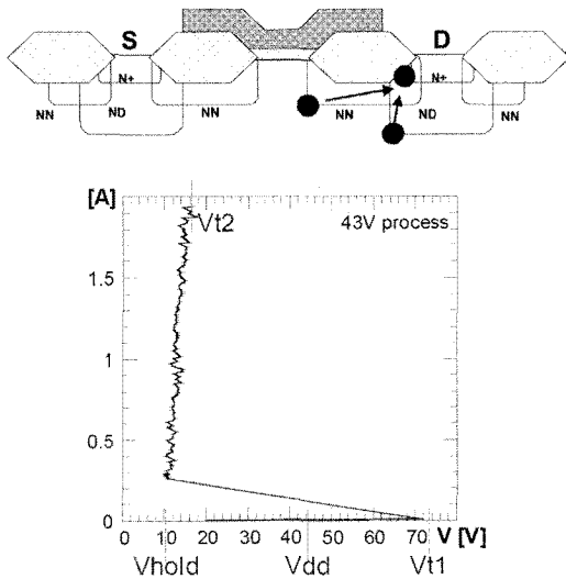
<그림 4> 고전압 MOSFET의 단면도 및 IV 특성
