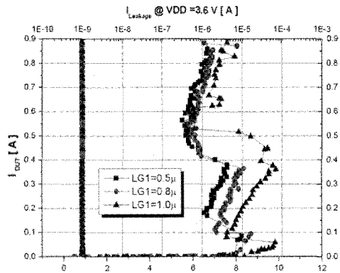
〈그림 7〉 PTSCR (P Substrate-Triggered SCR) 의 Layout 및 TLP-IV 특성
