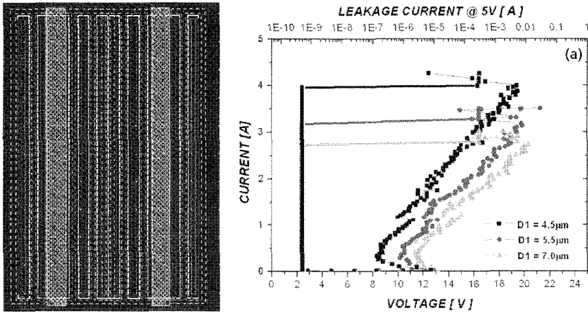
〈그림 8〉 HHVSCR(High Holding Voltage SCR)의 Layout 및 TLP-IV 특성
