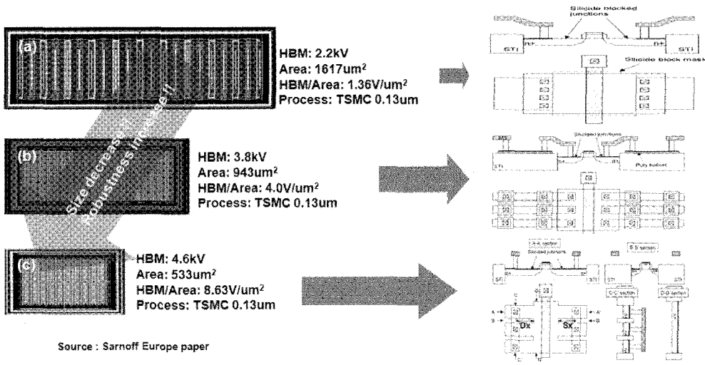
〈그림 6〉 (a) 일반적인 GGNMOS, (b) BEB(Back-End-Ballast) GGNMOS (c) AAS (Active Area Segmentation) GGNMOS
