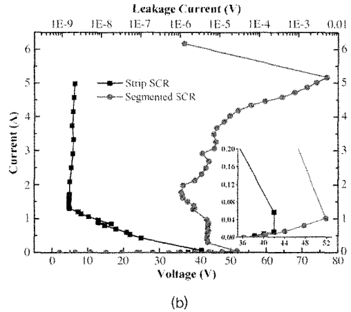
<그림 14> Segmented SCR의 (a)레이아웃, (b)TLP-IV 특성
