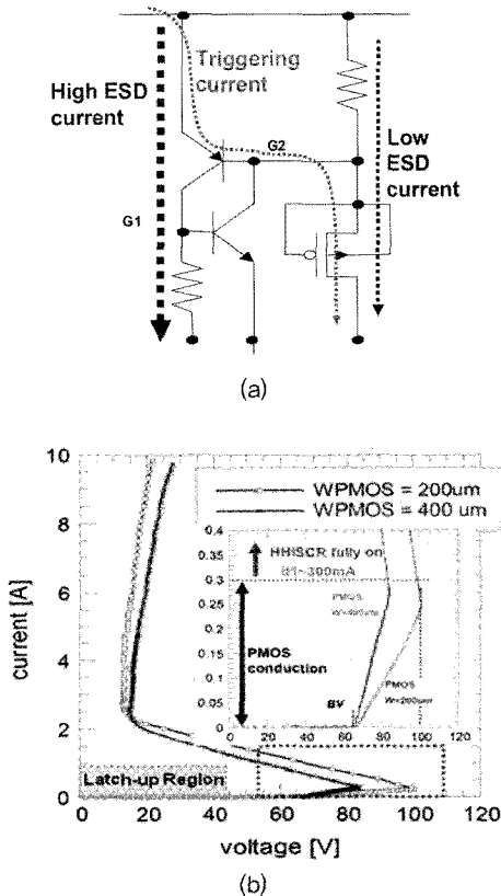
<그림 10> (a) PMOS Triggered SCR Power Clamp의 회로도, (b) TLP-IV 특성
