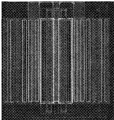
〈그림 7〉 PTSCR (P Substrate-Triggered SCR) 의 Layout 및 TLP-IV 특성
