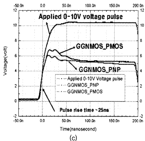
<그림 5> (a)바디 트리거 방식을 사용한 GGNMOS의 회로도, (b)TLP-IV 특성, (c) Turn-On 속도
