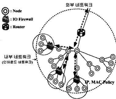
그림 3. IO 방화벽
