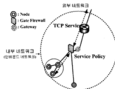
그림 1. Gate 방화벽
