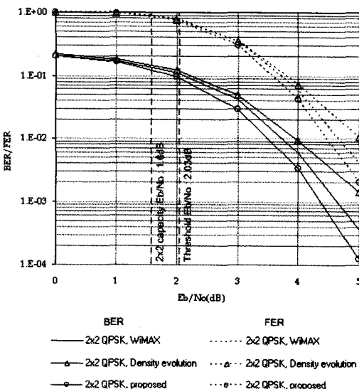
그림 4. 2x2 MAP detector 기반의 LDPC code 성능 곡선
