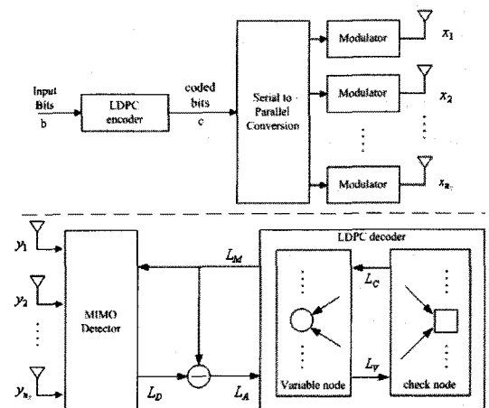
그림 1. 반복 복호를 사용하는 MIMO 기반의 LDPC code의 송수신기 구조
