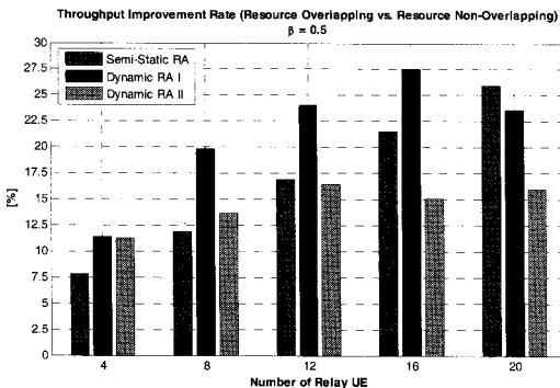
그림 16. 리소스 중복 할당 방식을 적용한 자원할당 기법의 평균 전송용량 증가율 비교 Fig. 16. Throughput improvement rate comparison of resource allocation schemes based on resource overlapping method
