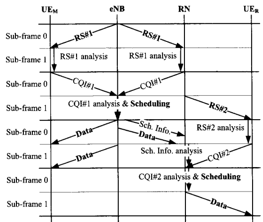
그림 4. 반정적 자원할당 기법을 위한 시그널링 흐름도 Fig. 4. Signaling flows of semi-static resource allocation scheme
