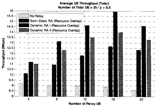
그림 15. 리소스 중복 할당 방식을 적용한 자원할당 기법의 평균 전송용량 성능 비교 Fig. 15. Average throughput performance comparison of resource allocation schemes based on resource overlapping method
