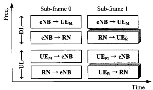
(b) 릴레이 기반의 시스템
