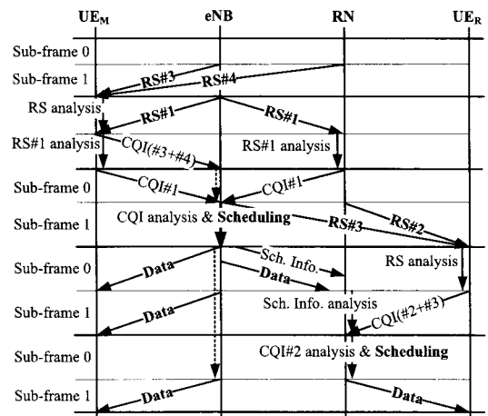
그림 10. 제안된 리소스 중복 할당 방식 기반의 반정적 자원할당 기법을 위한 시그널링 흐름도 Fig. 10. Signaling flows for semi-static resource allocation scheme based on the proposed overlapping method
