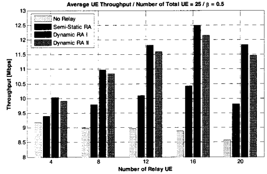
그림 14. 리소스 비중복 할당 방식을 적용한 자원할당 기법의 평균 전송용량 성능 비교 Fig. 14. Average throughput performance comparison of resource allocation schemes based on resource non-overlapping method
