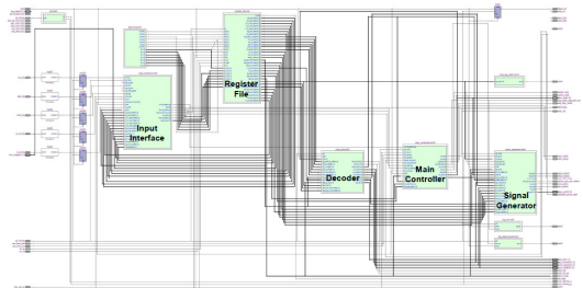
그림 13. TACAN FPGA의 전체 합성도 Fig. 13. Top synthesis result of TACAN FPGA
