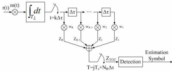
그림 2. 이산 시간 채널 모델에 대한 레이크 수신기. Fig. 2. RAKE receiver for discrete time channel model.
