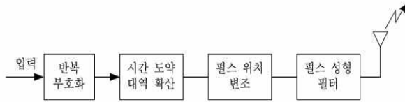
그림 1. 펄스 위치 변조-시간 도약 UWB 시스템 구조 Fig. 1. PPM-TH UWB system structure
