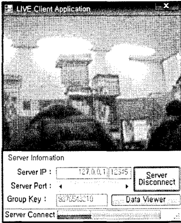
그림 7. 클라이언트
