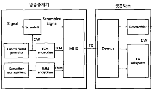
그림 1. CAS 시스템 구성도
