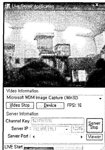
그림 6. 서버 송출부
