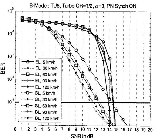
그림 11. 제안한 PN 기반 시간동기 방법의 BER
