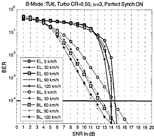
그림 9. 시간동기 오차가 없는 경우의 BER
