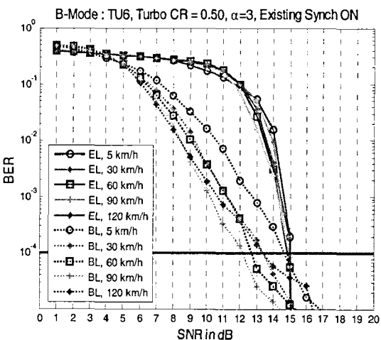
그림 10. 기존 시간동기 방법의 BER
