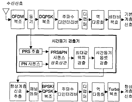
그림 7. 제안한 시간동기 블록도
