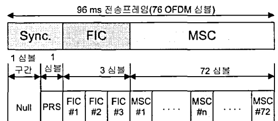
그림 4. AT-DMB 데이터 프레임 구조
