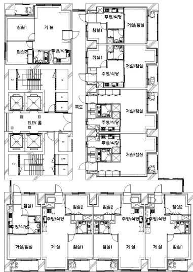
그림 4. 평면도
