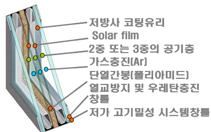
그림 1. 단열창호 슈퍼윈도우의 개념도
