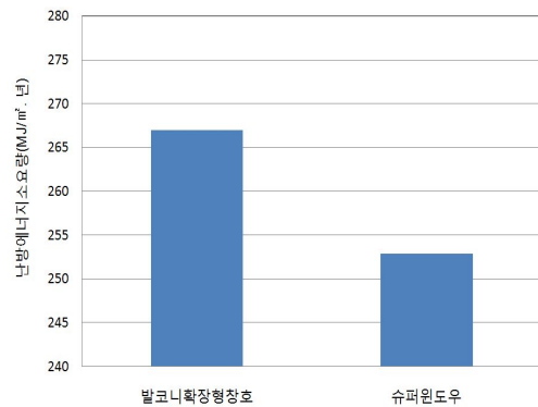
그림 5. 난방에너지소요량
