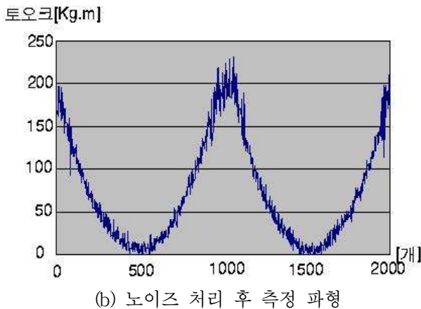
그림 10 노이즈 처리 전, 후의 파형 비교
