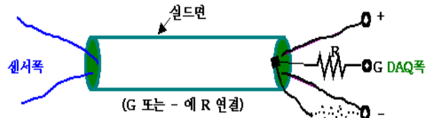
그림 8 저항 삽입 방법
