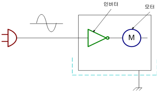
(b) 케이스 실드 (Case Shield)
