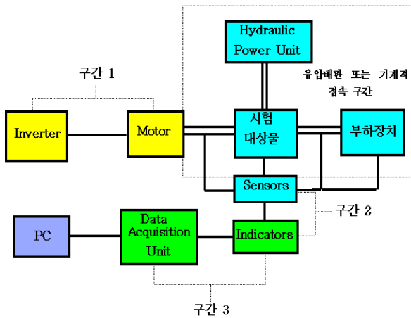
그림 2 유압 시험장비의 노이즈 대책 구간
