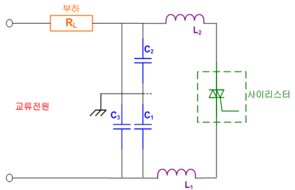
(b) 2선 필터
