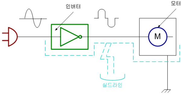
(a) 라인실드 (Line Shield)
