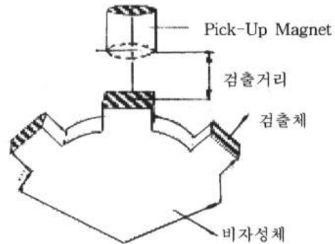
(b) 펄스방식 센서의 원리
