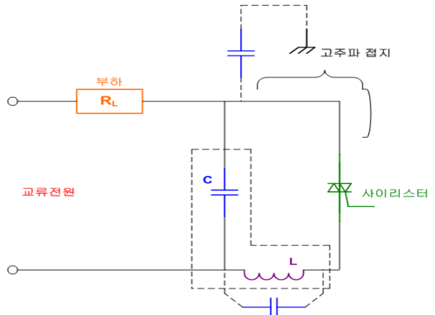
(a) 1선 필터
