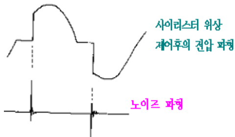
그림 1 사이리스터(Thyristor)에 의한 노이즈
