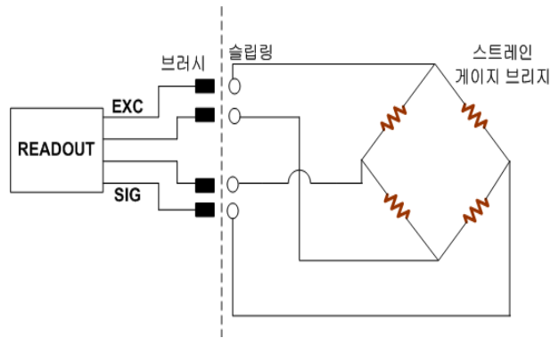
(a) 브리지방식 센서의 원리
