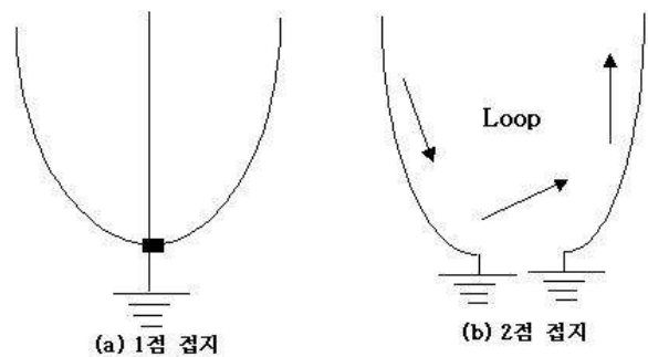
그림 3 접지(Ground) 방법
