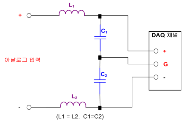
그림 9 로우-하이 필터(Low+High Filter)
