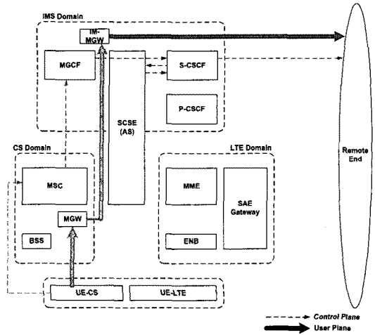
그림 7. CS망에서의 호 설정 Fig. 7. CS originating call
