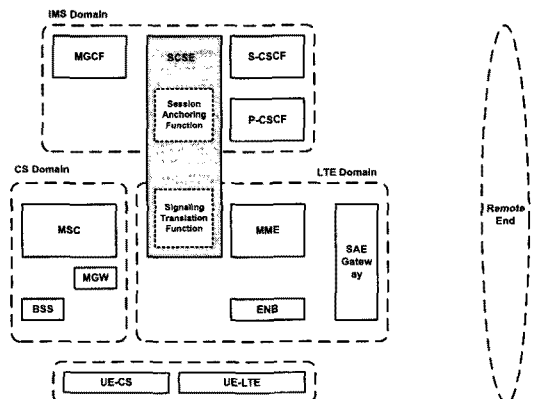
그림 4. SCSE 구조도 Fig. 4. SCSE architecture
