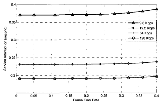
그림 13. CS망의 라디오링크 상황에 따른 서비스 장애 발생시간 : LTE망에서 CS망으로의 핸드오버 Fig. 13. Service interruption time according to radio link condition of CS network : LTE to CS handover
