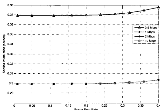
그림 14. LTE망의 라디오링크 상황에 따른 서비스 장애 발생시간 : CS망에서 LTE망으로의 핸드오버 Fig. 14. Service interruption time according to radio link condition of LTE network : CS to LTE handover
