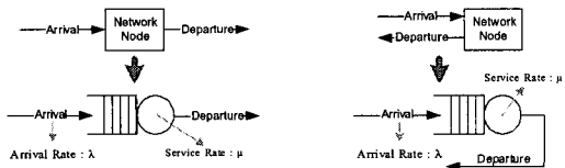
그림 9. M/M/1 큐잉 모델 Fig. 9. M/M/1 queueing model
