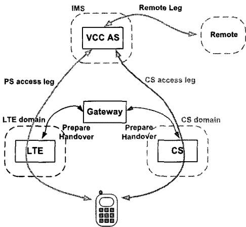
그림 3. 게이트웨이 방법 Fig. 3. Gateway approach
