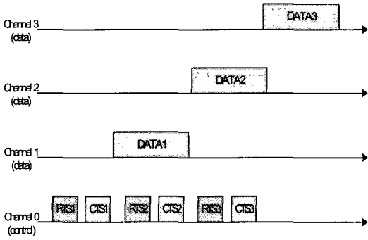
(a) 2개의 인터페이스를 사용하는 single rendezvous 프로토콜
