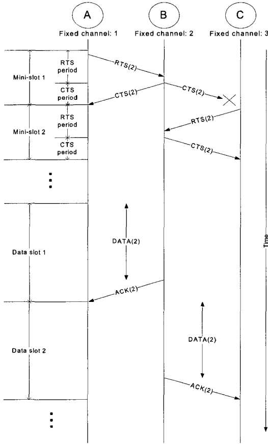
그림 9. 멀티채널 히든 노드 문제를 해결하는 예
