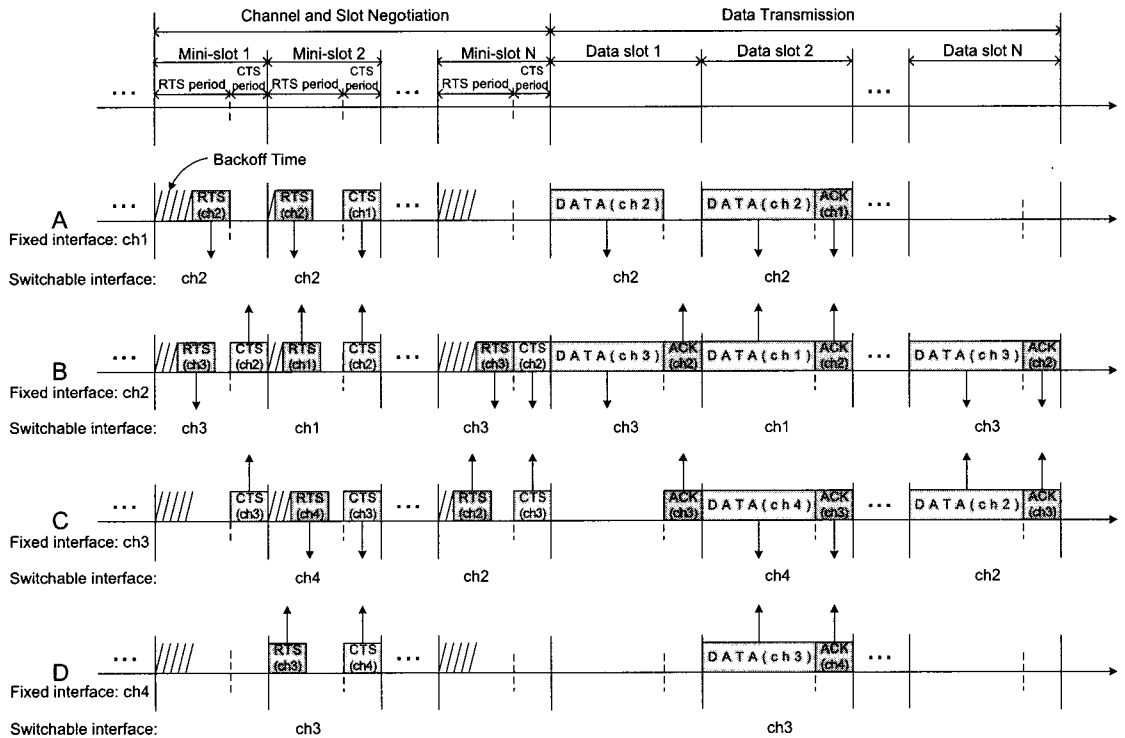
그림 8. 제안한 MAC 프로토콜의 동작 예
