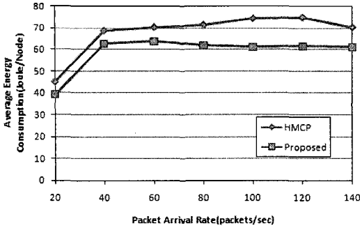
그림 14. 노드 당 평균 에너지 소비
