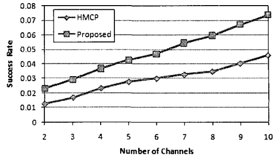
그림 12. 채널수에 따른 데이터 전송 성공률
