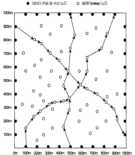
그림 10. 모의실험 토폴로지
