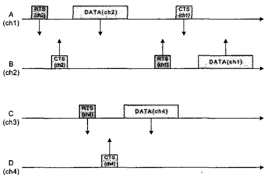
(b) 1개의 인터페이스를 사용하는 multiple rendezvous 프로토콜
