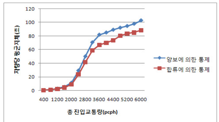
좌 : 직 : 우 = 1 : 4 : 8
