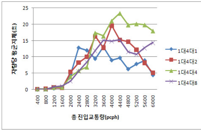
방식에 따른 차량당 평균지체 차이
