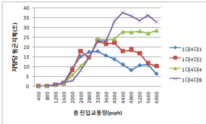
설치 전·후 차량당 평균지체 차이
