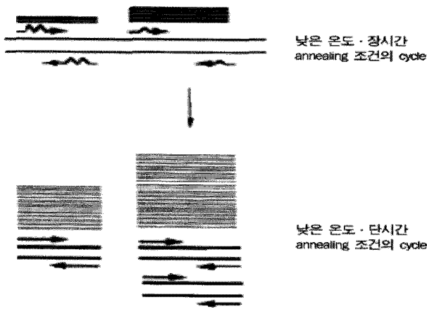
Fig. 3. AP-PCR 원리. 자료 : Okano 등 (2002) 38) .
