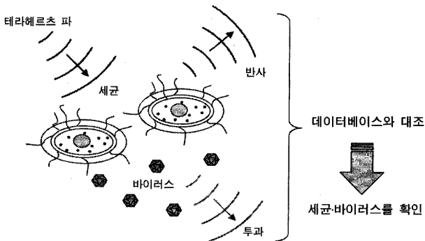
Fig. 5. 테라헤르츠 분광/영상의 세균 검사에의 응용. 자료 : 전 등 (2009) 45) .
