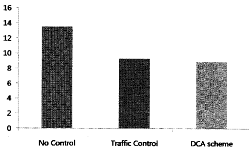
그림 9. 각 기법의 패킷 손실률 비교
