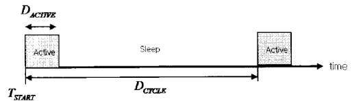
그림 2. 듀티사이클 파라미터
