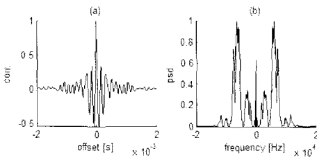
그림 10. 대표적인 손가락딱소리의 (a) 상관함수 (b) 전력스펙트럼밀도
