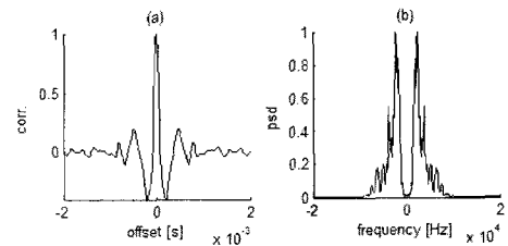
그림 7. 대표적인 A형 박수소리 (a) 상관함수 (b) 전력스펙트럼밀도
