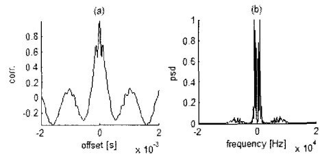
그림 8. 대표적인 B형 박수소리의 (a) 상관함수 (b) 전력스펙트럼밀도
