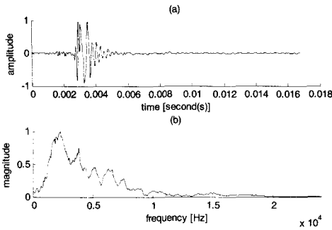
그림 2. 대표적인 A형 박수소리 (a) 시간영역 (b) 주파수영역
