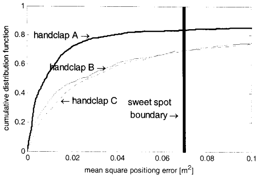
그림 21. 반향이 있는 일반공간에서 박수소리를 측위음으로 사용했을 때 평균자승측위오차의 누적분포함수
