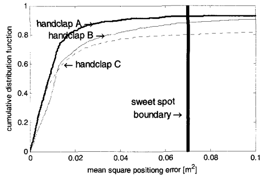
그림 19. 무반향실에서 박수소리를 측위음원으로 사용했을 때 평균자승측위오차의 누적분포함수
