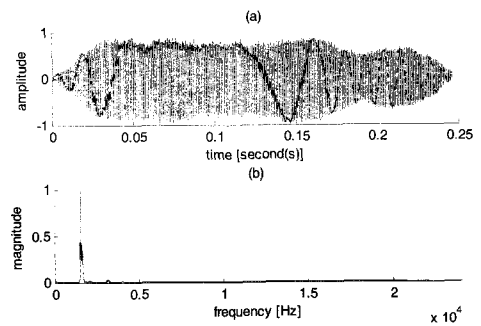
그림 6. 대표적인 휘파람소리 (a) 시간영역 (b) 주파수영역
