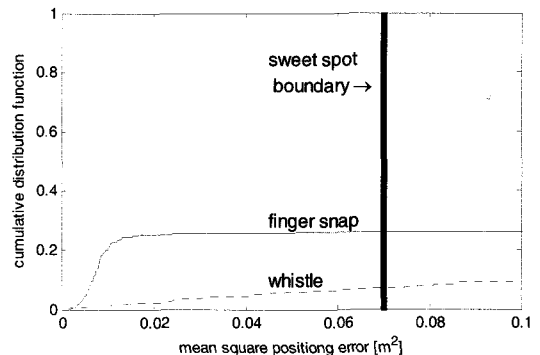
그림 20. 무반향실에서 손가락소리와 휘파람소리를 측위음원으로 사용했을 때 평균자승측위오차의 누적분포함수
