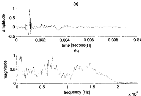
그림 4. 대표적인 C형 박수소리 (a) 시간영역 (b) 주파수영역
