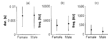
그림 15. 성별에 따른 손가락딱소리의 (a) 초과지연시간, (b) 최대주파수, (c) 대역폭의 평균과 분산
