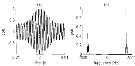
그림 11. 대표적인 휘파람소리의 (a) 상관함수 (b) 전력스펙트럼밀도
