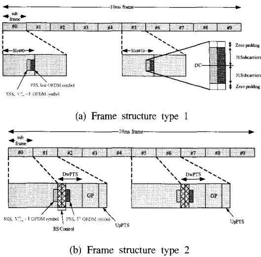
그림 1. LTE 시스템의 프레임 구조
