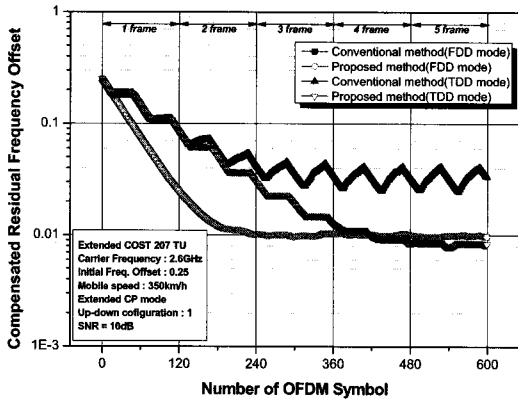
그림 10. Tracking 성능 비교[Proposed method vs. Conventional method]
