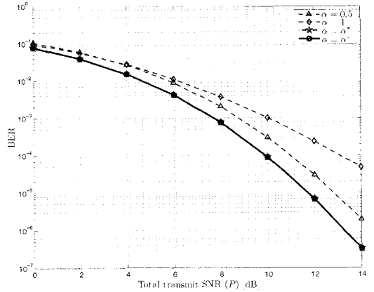
그림 3. ( \sigma_{SD}^2, \sigma_{SR}^2, \sigma_{RD}^2 ) = (1, 1, 4)인 비대칭 레일리 페이딩 채널에서 전력 분배비 \alpha = 0.25, 0.5, 1, \alpha_a^*, \alpha_a^* 에 대한 SDF 방식의 비트 오류율 비교
