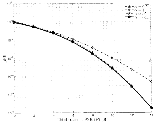
그림 4. ( \sigma_{SD}^2, \sigma_{SR}^2, \sigma_{RD}^2 ) = (1, 4, 1)인 비대칭 레일리 페이딩 채널에서 전력 분배비 \alpha = 0.25, 0.5, 1, \alpha_a^*, \alpha_a^* 에 대한 SDF 방식의 비트 오류율 비교
