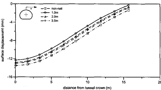
그림 9. 네일 간격변화에 따른 지표침하
