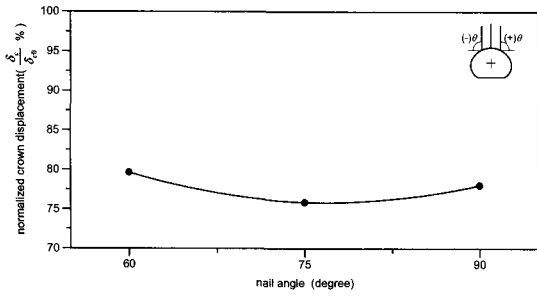
그림 12. 네일 설치각도변화에 따른 정규화 천단침하
