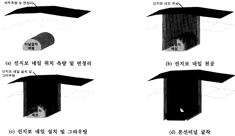
그림 5. PNT공법 시공순서
