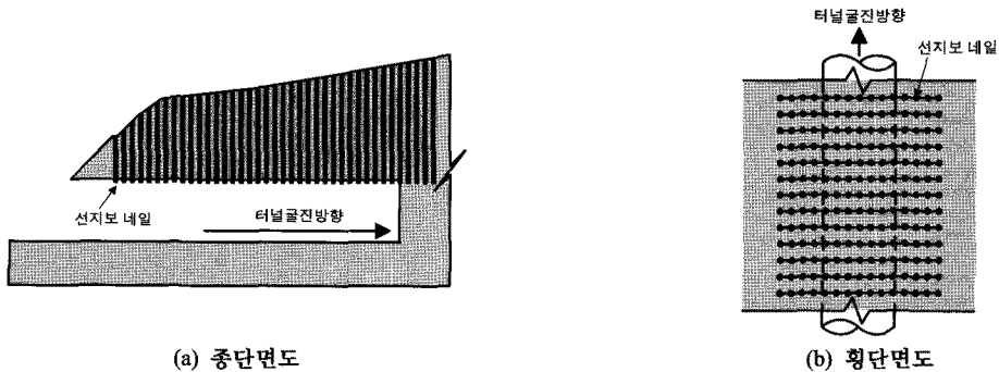
그림 1. PNT공법 개요도
