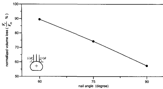
그림 15. 네일 설치각도변화에 따른 체적손실
