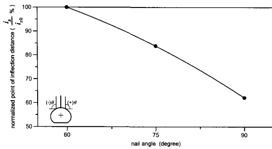
그림 14. 네일 설치각도변화에 따른 변곡점( i_x )변화
