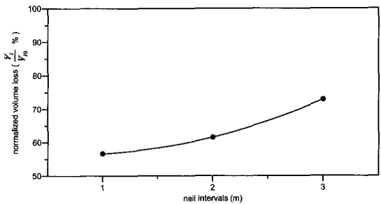
그림 11. 네일 간격변화에 정규화 체적손실
