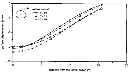
그림 13. 네일 설치각도변화에 따른 지표침하
