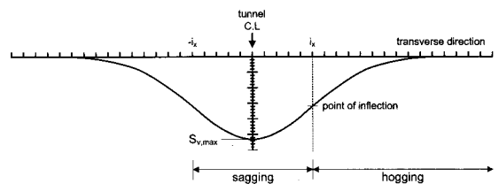
그림 7. 횡방향 침하형상(Franzius, 2003)
