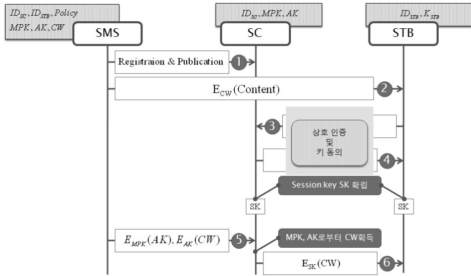
(그림 3) McCormac Hack 공격을 막기 위한 SC와 STB간 키 동의
