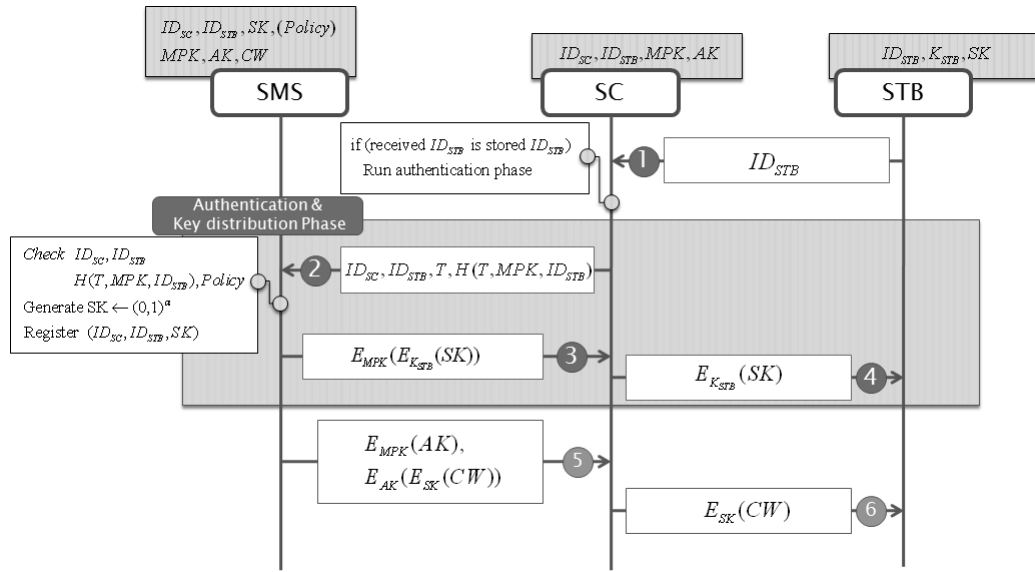
(그림 8) 제안하는 SC-STB 인증 프로토콜
