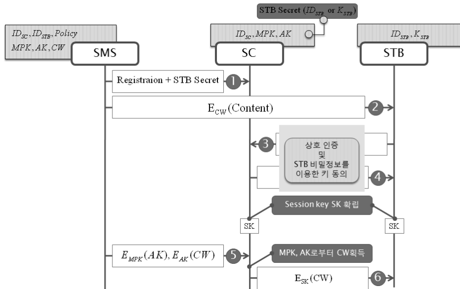
(그림 4) SC복제를 위한 SC와 STB의 바인딩
