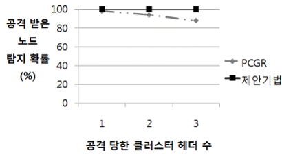
(그림 10) CH가 키 정보를 줄 경우 공격을 감지할 확률
