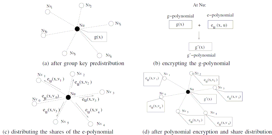
(그림 1) PCGR기법의 그룹 초기화
