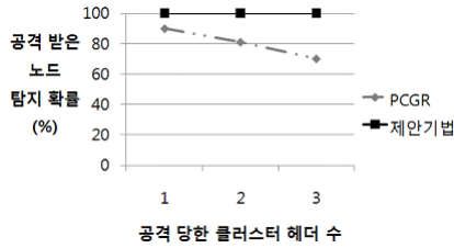
(그림 11) CH가 키 정보를 주지 않을 경우, 또는 감지를 피하기 위해 정확한 값을 주는 경우 공격을 감지할 확률
