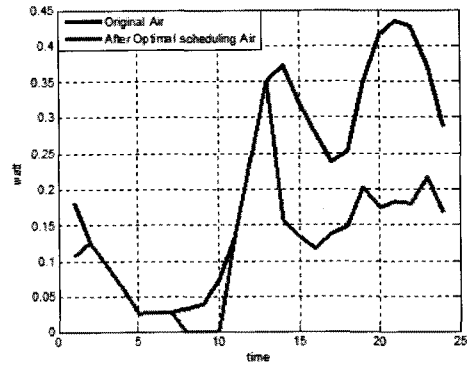
그림 11. 에어컨 사용 패턴 함수 결과 그래프
