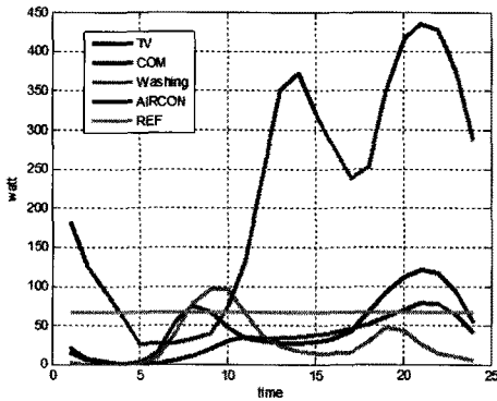
그림 7. 5종류의 가정용 전력 기계의 capacity를 고려한 사용패턴 함수
