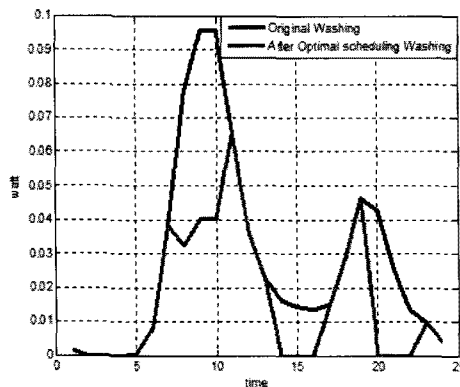
그림 10. 세탁기 사용 패턴 함수 결과 그래프
