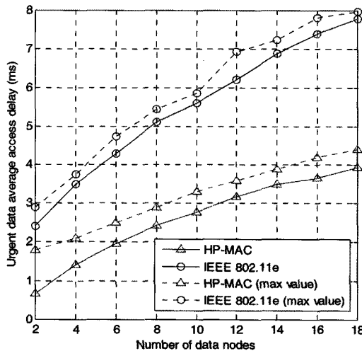
그림 7. 여러 개의 데이터 노드들을 통한 긴급 데이터 접근 지연 Fig. 7. Urgent data access delay by number of data nodes
