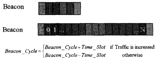
그림 3.1. 비컨 싸이클 Fig. 3.1. Beacon Cycle
