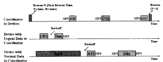
그림 1. 우선순위 전송 Fig. 1. Priority Transmission
