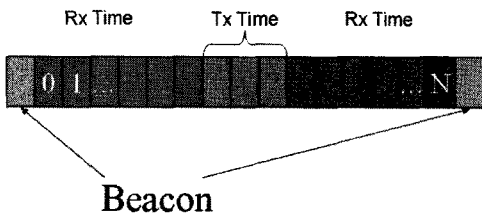
그림 2. 비컨 구조 Fig. 2. Beacon Structure
