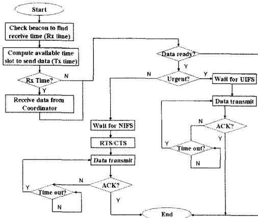
그림 5. 디바이스 전송 플로우 차트 Fig. 5. Device Transmission Flow Chart
