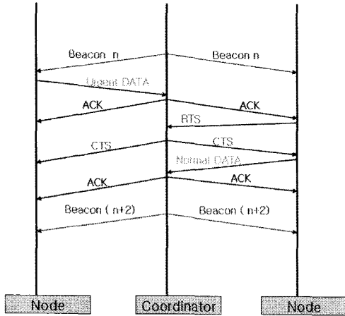
그림 4. 한 개의 비컨 사이클 전송 Fig. 4. One Beacon Cycle Transmission
