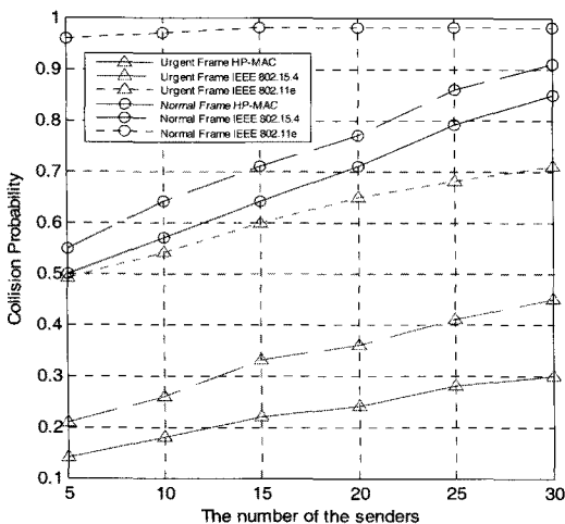
그림 10. 송신 노드 수에 따른 충돌 발생률 Fig. 10. Collision by number of senders
