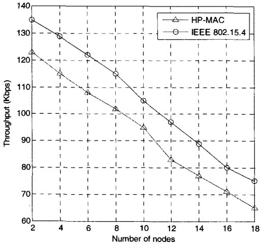
그림 9. 노드 수에 따른 처리량 비교 Fig. 9. Throughput by number of nodes
