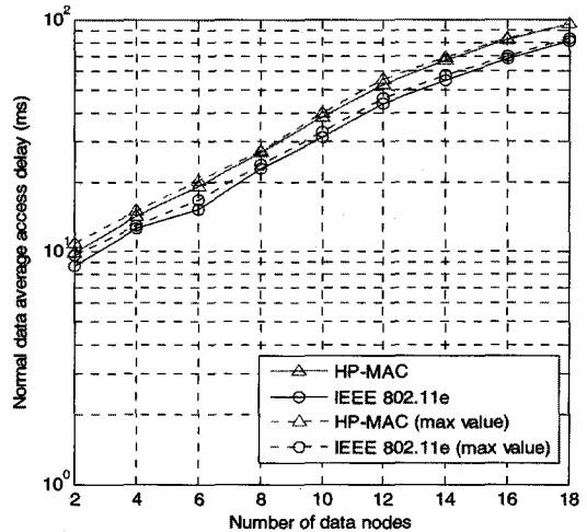
그림 8. 다수의 데이터 노드들에 의한 일반 데이터 접근 지연 Fig. 8. Normal data access delay by number of data nodes
