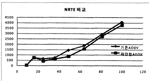
그림 10. NRTE 비교
