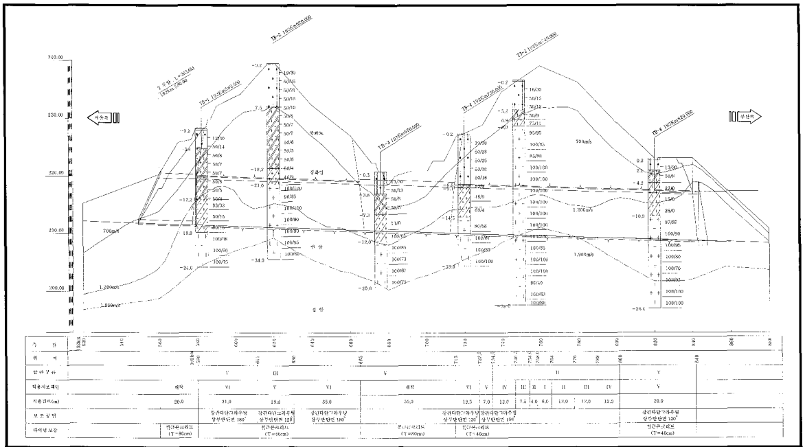
그림 5. OO터널 지층단면 및 지보패턴적용현황
