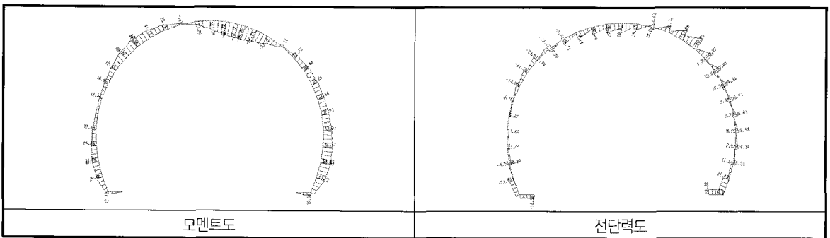
그림 9. 인버트 폐합전의 단면력도
