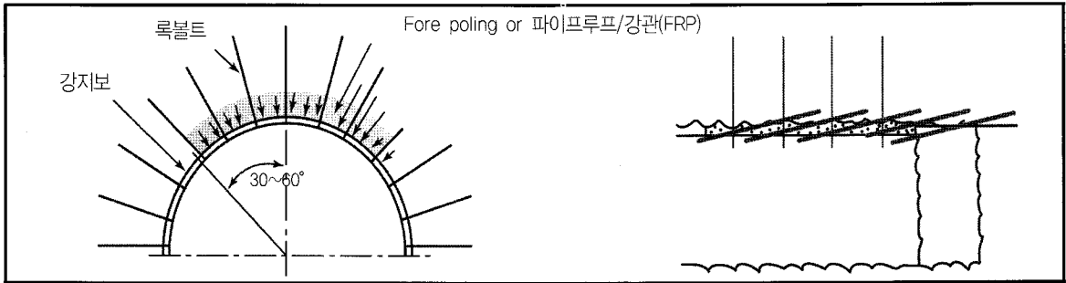
그림 2. Fore-Poling, 파이프루프/강관(FRP) 설치개념도
