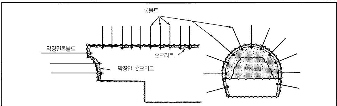
그림 4. 막장면 안정대책 설치개념도
