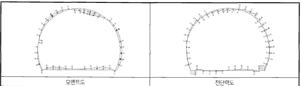
그림 10. 인버트 폐합후의 단면력도
