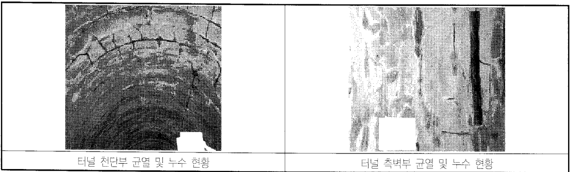
그림 7. △△터널 변형 사진
