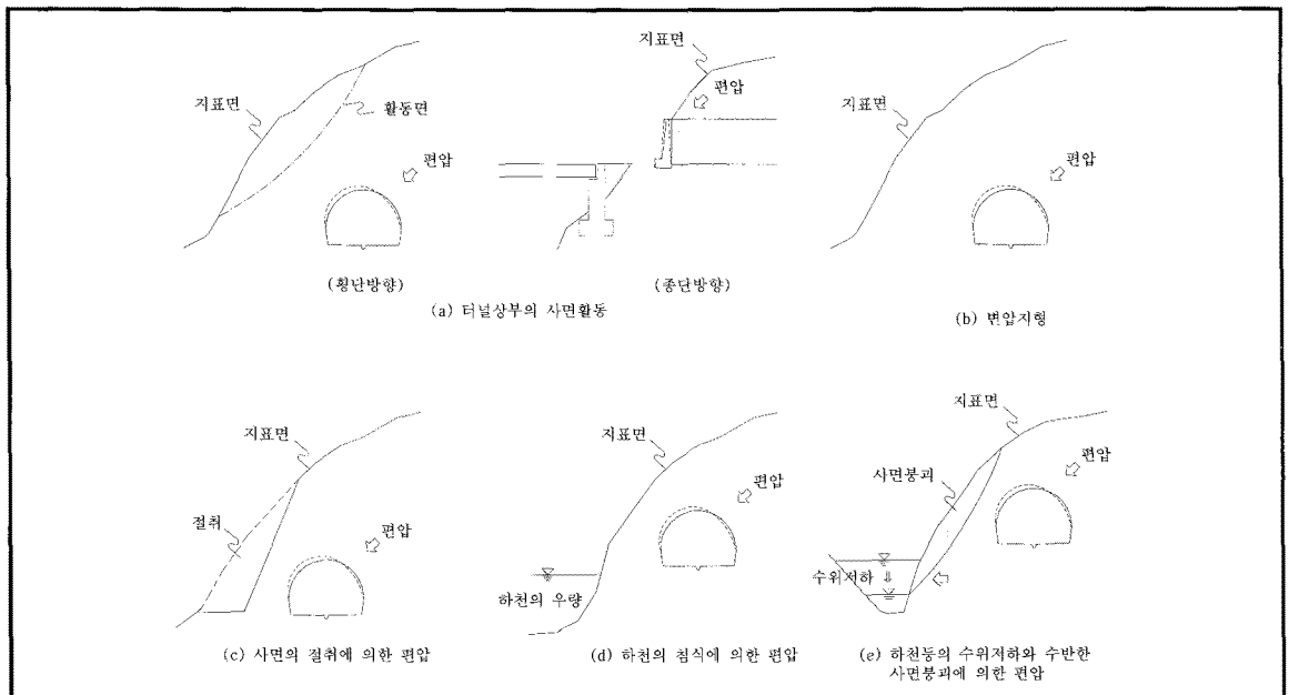
그림 1. 저토피·편경사지형의 터널거동
