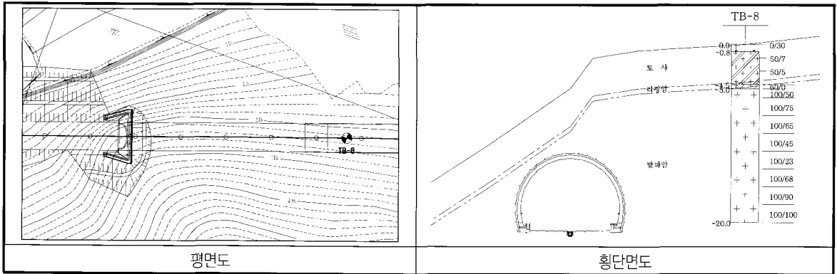
그림 8. 검토단면 현황도
