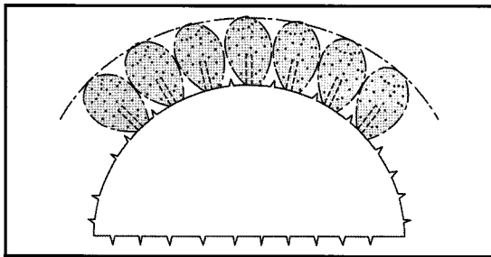
그림 3. 그라우팅 공법 설치개념도
