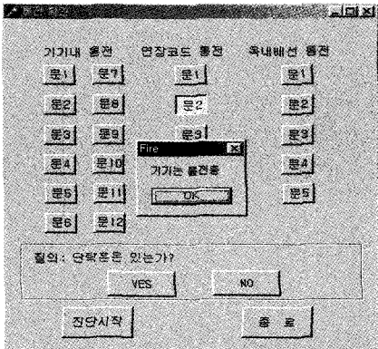
[그림 7] 통전상태 진단 창
