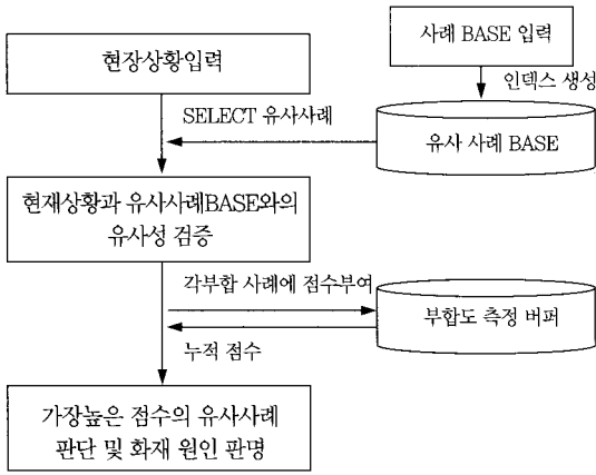
[그림 5] 사례기반 추론 과정
