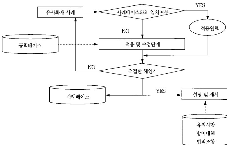
[그림 6] 해의 적응, 수정 및 학습과정
