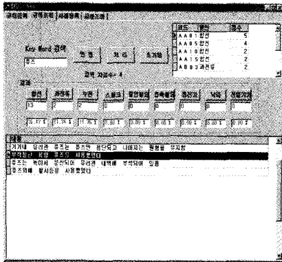
[그림 13] 규칙기반 추론 결과
