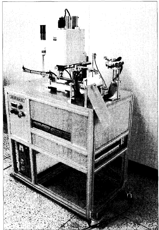
초음파를 이용한 Auto Gate Cutting M/C
