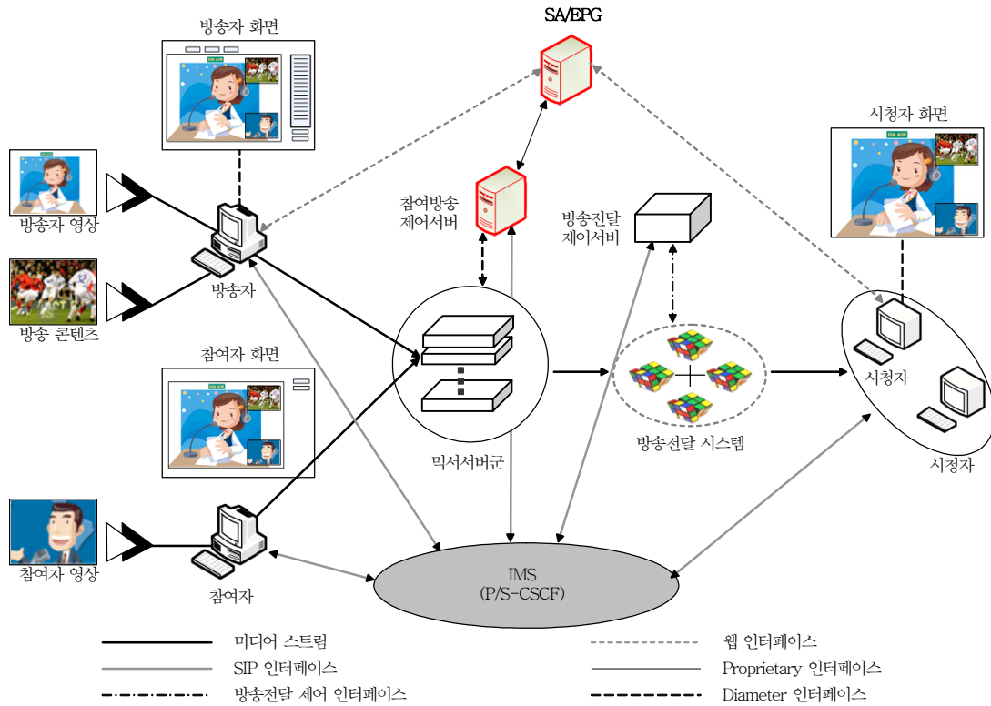
(그림 2) IMS 연동형 IPTV 참여형방송 시스템 구조
