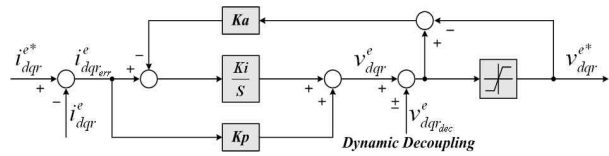
그림 1 이중여자자유도 풍력발전기의 회전자측 전류제어기 Fig. 1 current controller of RSC for DFIG
