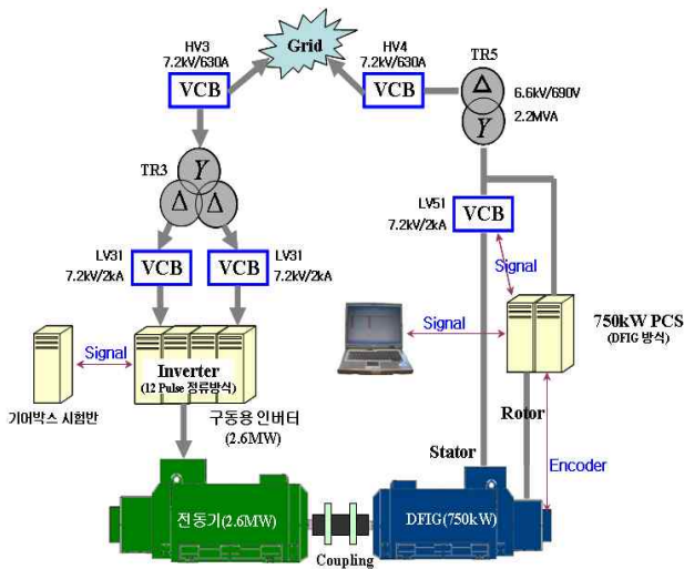
그림 9 2MW급 DFIG 시스템 시험장치 구성 Fig. 9 configuration of 2MW DFIG test setup for 2MW class DFIG system
