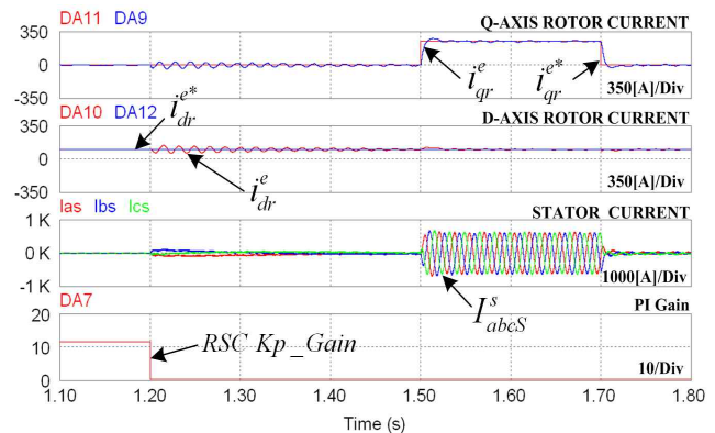
그림 5 가변 PI 이득 값을 적용한 회전자 전류제어 Fig. 5 RSC current control using variable PI gains
