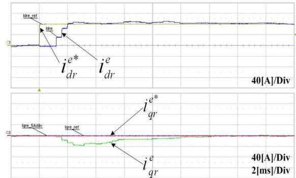
그림 8 회전자 가변 전류제어 이득 값을 적용한 DFIG의 동특성 Fig. 8 dynamic performance of DFIG rotor current controller using variable PI controller gain
