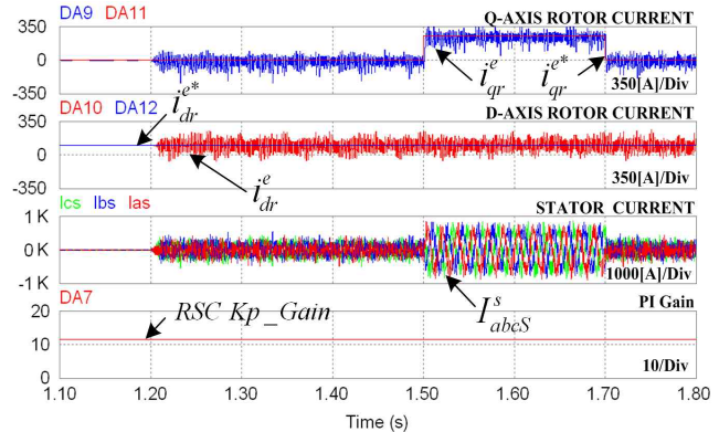
그림 4 고정 PI 이득값을 적용한 회전자 전류제어 Fig. 4 RSC current control using constant PI gain
