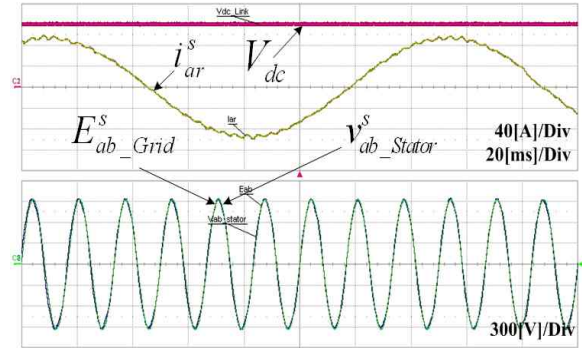
그림 7 회전자 가변 전류제어 이득 값을 적용한 DFIG의 계통연계시 운전특성 Fig. 7 grid connected operation of DFIG using rotor variable PI controller gain
