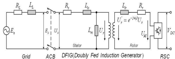
그림 2 이중여자 풍력발전기의 계통연계 등가회로 Fig. 2 grid connection equivalent circuit of the DFIG
