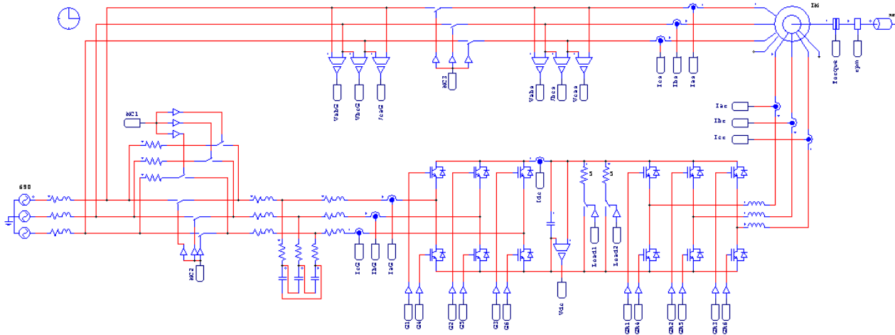
그림 3 이중여자유도 풍력발전기의 시뮬레이션 모델 Fig. 3 simulation model for DFIG system
