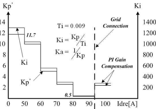
그림 6 발전기 인덕턴스 변화를 고려한 DFIG 회전자 전류제어기 가변이득 Fig. 6 variable gain of DFIG rotor current controller considering generator inductance variations
