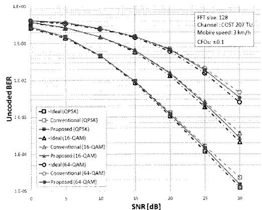
그림 8. 변조 차수에 따른 BER 성능 비교 (CFOs = \pm 0.1 )
