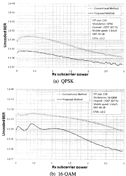
그림 7. 기존 방식과 제안하는 방식의 수신 부반송파 전력에 따른 초기 추정 오류 비교
