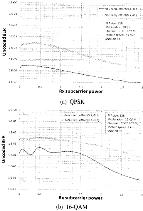
그림 6. 기존의 반복적 ICI 제거 기법의 수신 부반송파 전력에 따른 초기 추정 오류
