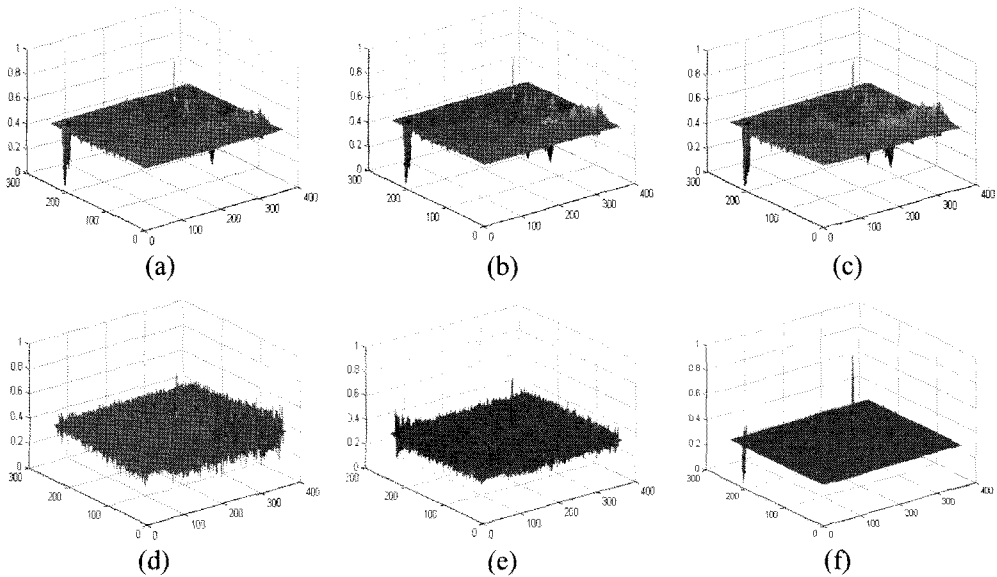
그림 6. 영상 D1에 대한 (a) Median 11×11, (b) Median 9×9, (c) Median 7×7, (d) TDLMS, (e) TDNLMS, 및 (f) 제안한 방법에 의한 결과 영상
