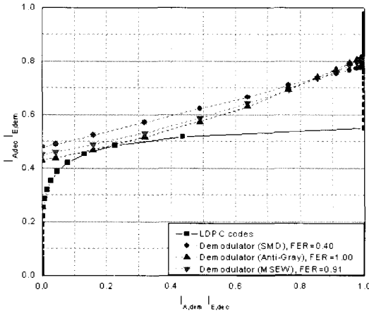
그림 9. 복조기와 복호기 간의 부가 정보 교환을 나타내는 EXIT 도표 (다양한 맵핑)
