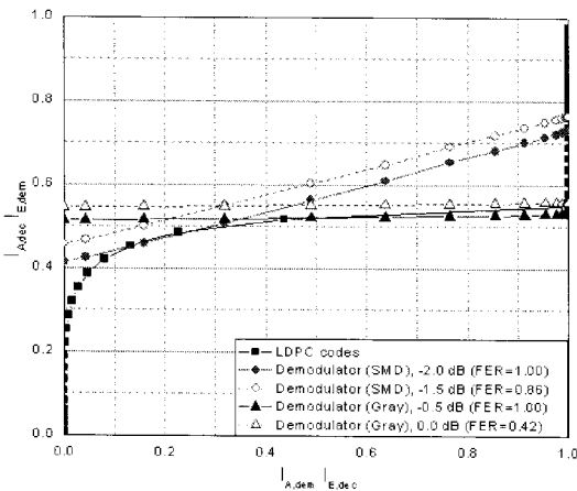
그림 7. 복조기와 복호기 간의 부가 정보 교환을 나타내는 EXIT 도표
