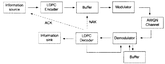
그림 1. 시스템 모델
