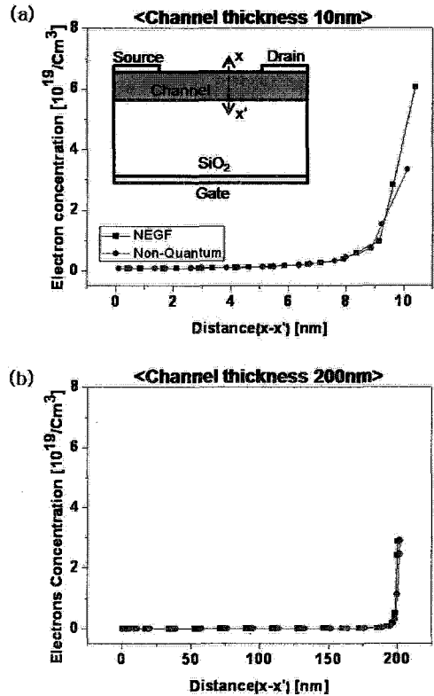
그림 5. 양자 모델을 적용한 전자 농도 분포도. (a) 채널의 두께가 10 nm, (b) 채널의 두께가 200 nm Fig. 5. Electrons concentration distribution graph by the quantum model. (a) Channel Thickness 10 nm, (b) Channel Thickness 200 nm
