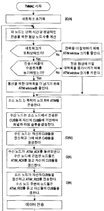
그림 3. TMMAC의 작동과 복잡도 계산
