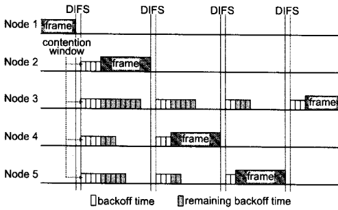
그림 3. DCF에서의 백오프 절차
