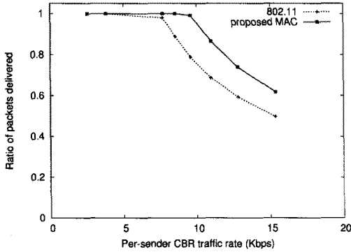
그림 9. CBR 트래픽에서 센서 노드들의 패킷 전송률
