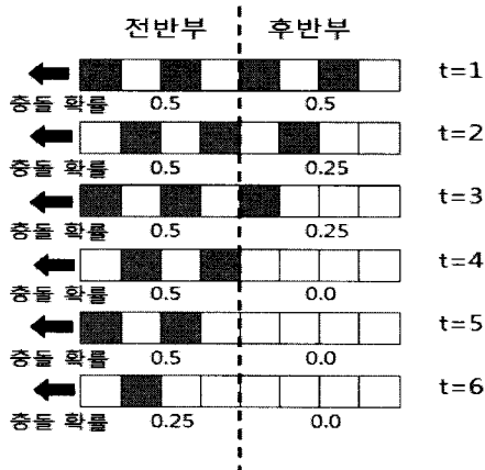
그림 1. IEEE 802.11에서 DCF를 이용한 접근 방식
