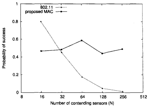
그림 7. 센서 수(N)에 따른 전송확률( p=0.6, CW=32 )
